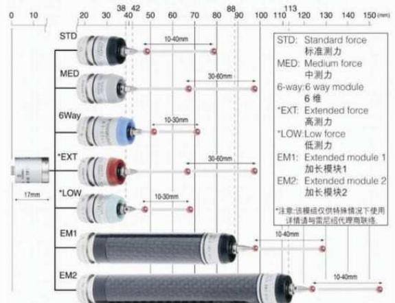
各模块的测针建议使用长度如下:
