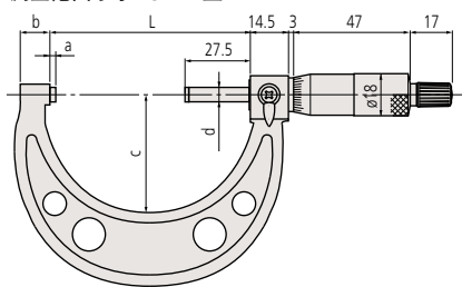
测量范围小于 75mm 型
