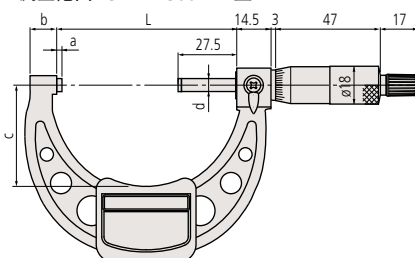
测量范围 75mm - 300mm 型
